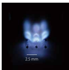
マイクロバーナアレイ(ノズル径70μm)に形成された火炎
