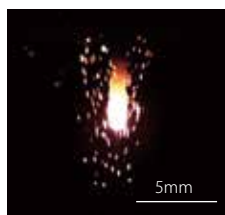
微小拡散火炎群による無機材料の積層造形の様子
