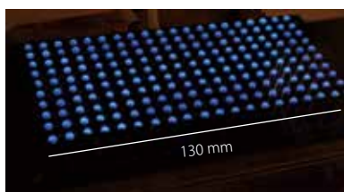
マイクロバーナアレイ(ノズル径0.7mm)に形成された微小拡散火炎
